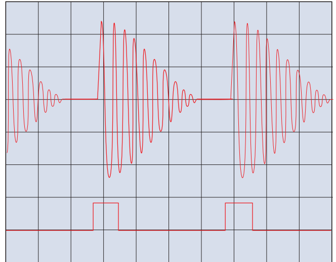
Bild 4: getriggertes Arbitrary-Signal
